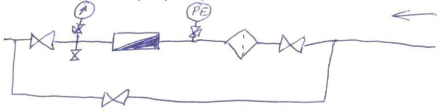
Схема узла учета (условные обозначения выполнены согласно ГОСТ)
